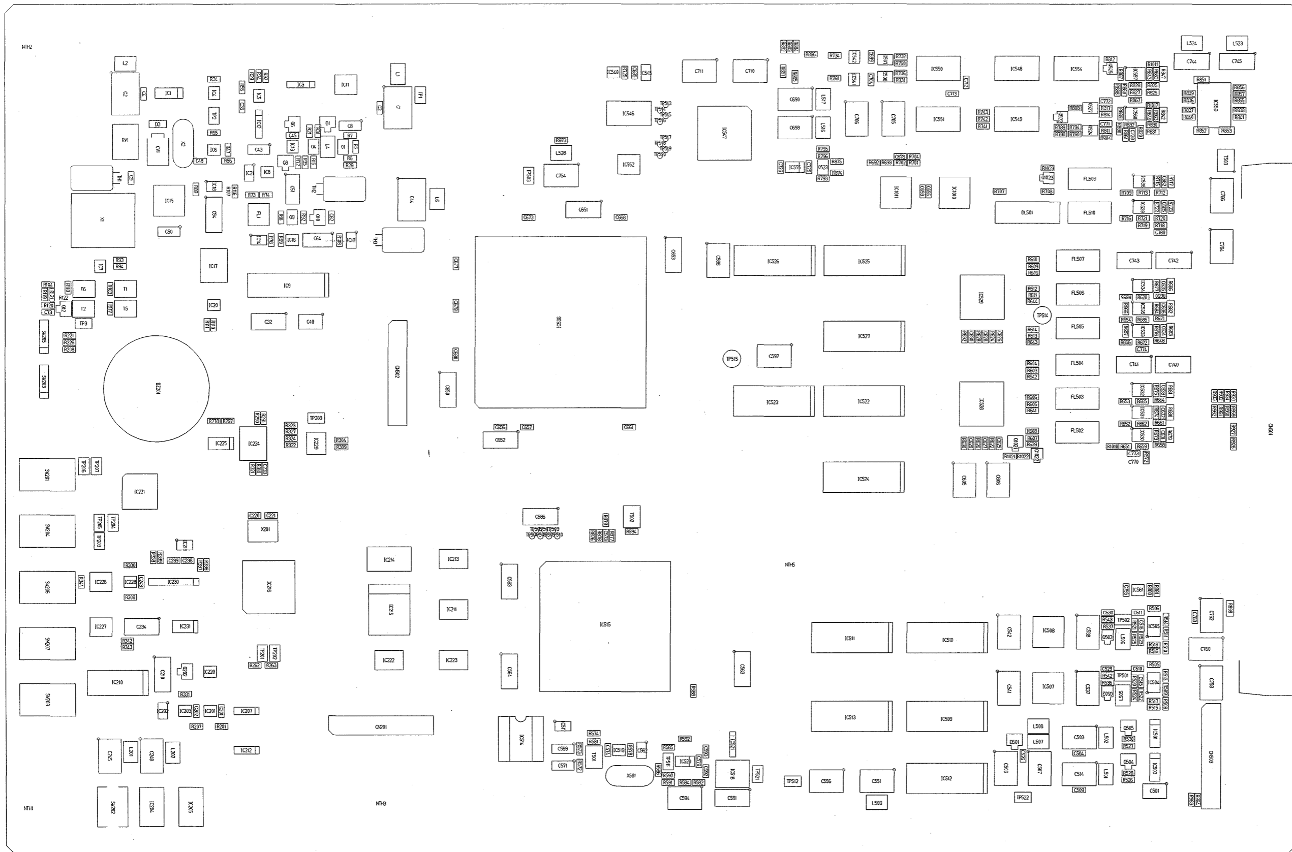
TU-VIDEO(PT-1518D) SIDE A
